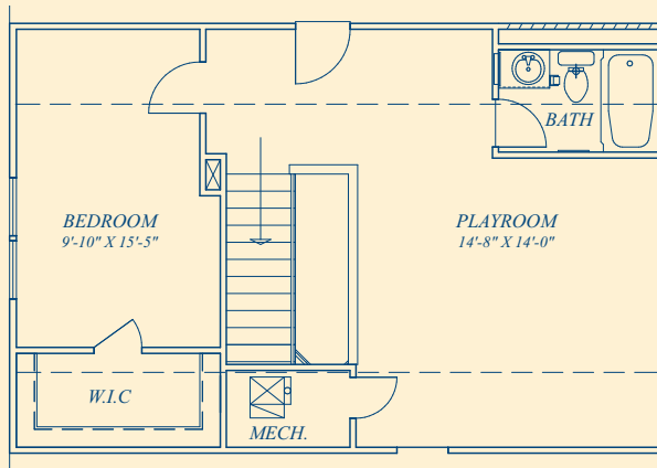
OPT. LOFT FLOORPLAN**
